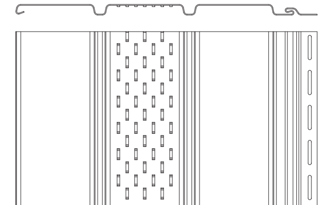
Panel wentylacyjny (perforowany)
